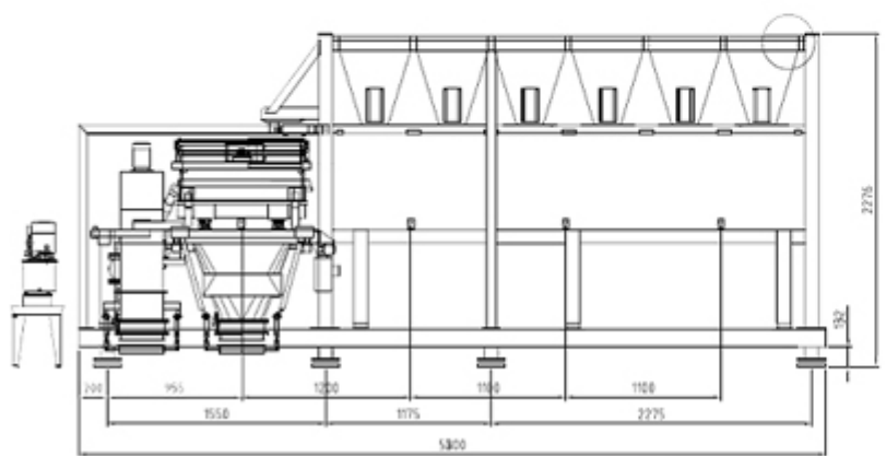
ALFRA自動計量システムFCD 2 4外形図
