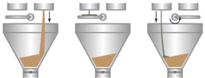
①メインスケールによる大容量計量(100Kg/B) ②サブスケールによる微量計量(5Kg/B) ③サブスケール反転払い出し
